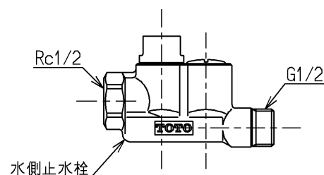
水側止水栓
