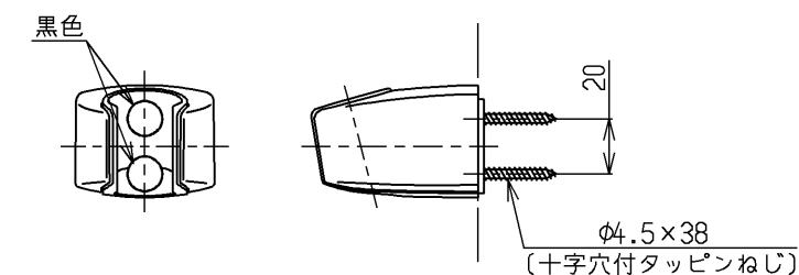
シャワーハンガー（2ヶ）
